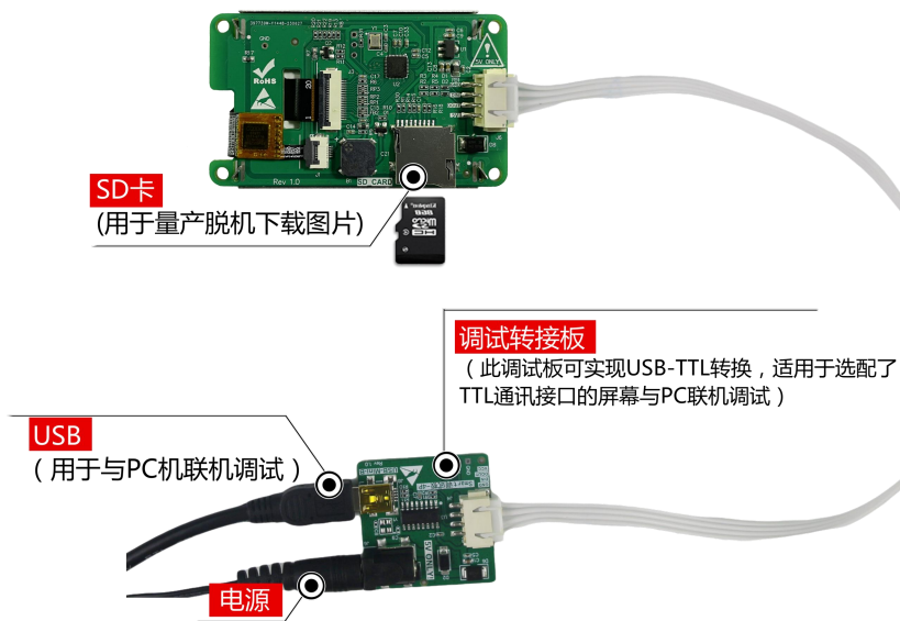
图 1-4 调试工具图
