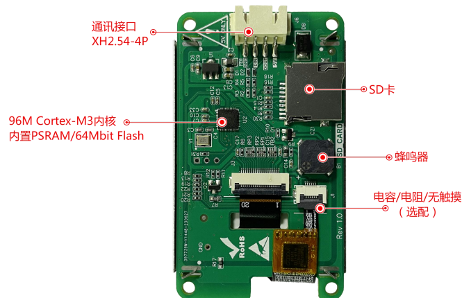
图 1-3 硬件配置图
